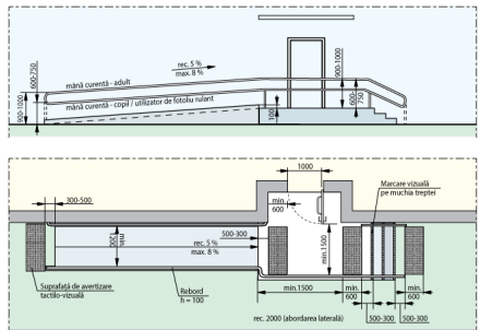
Fig. V.32.b Rampă de acces paralelă cu intrare în clădire
