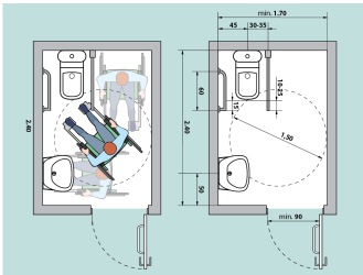
Fig. V.43.a Amplasarea unei cabine WC adaptate - tip B
