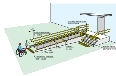
Fig. V.31.a Rampă de acces perpendiculară cu intrare în clădire
