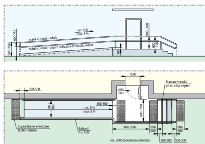
Fig. V.32.h Pământ de acces paralelă cu intrare în clădire
