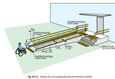
Fig. V.31.a Rampă de acces perpendiculară pe intrarea în clădire
