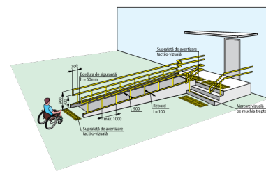
Fig. V.31.a Pantă de acces perpendiculară pe intrare în clădire
