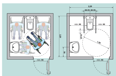
Fig. V.42.a Amplasarea unei cabine WC adaptate - tip A
