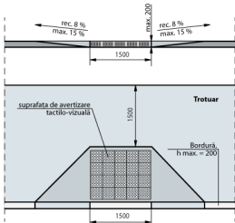
Fig. IV.9 Rampă de acces între trotuar și carosabil
