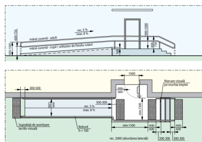
Fig. V.32.b Pămă de acces paralelă cu intrare în clădire
