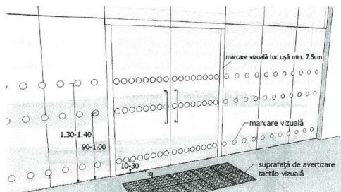
Fig. V.24. – Exemplu de conformare a suprafețelor vitrate în cadrul foi de ușă și realizarea contrastului vizual, atunci când ușa și suprafețele adiacente sunt vitrate
