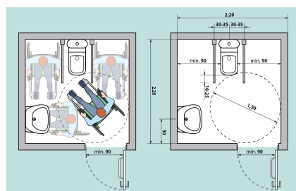
Fig. V.42a Amplasarea unei cabine WC adaptate - tip A
