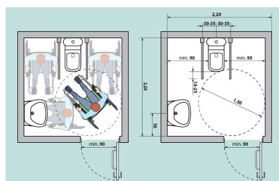
Fig. V.42.a Amenajarea unei cabină WC adaptate - tip A
