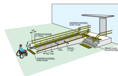
Fig. V.31.a Ramoă de acces perpendiculară pe intrarea în clădire
