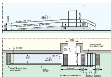
Fig. V.32.b Ramă de acces paralelă cu intrare în clădire
