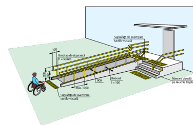
Fig. V.31.a Rămpă de acces perpendiculară pe intrarea în clădire
