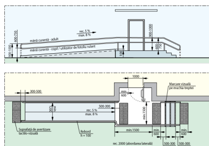
Fig. V.32.b Părpă de acces paralelă cu intrare în clădire
