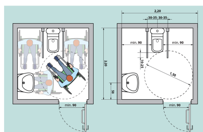
Fig. V42a Amenajarea unei cabină WC adaptate - tip A
